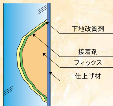
●F-4 工法施工図
