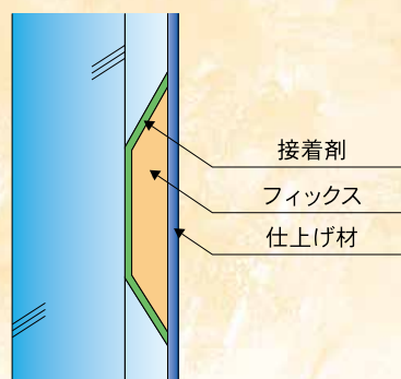
●F-2 工法施工図
