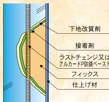
●F-3 工法施工図
