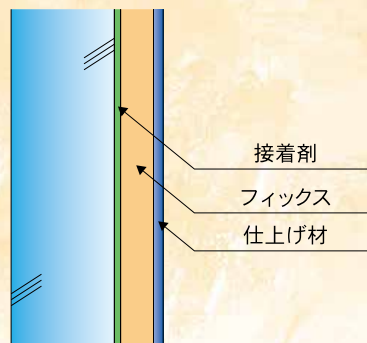
●F-1 工法施工図
